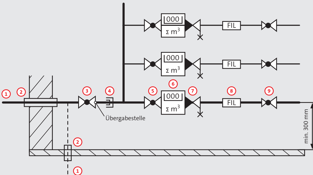
Abbildung 1: ein Zählerplatz
